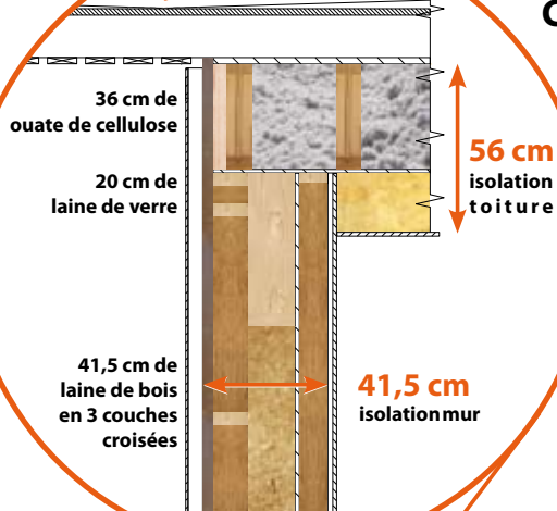
Coupe verticale de la jonction mur / toiture
